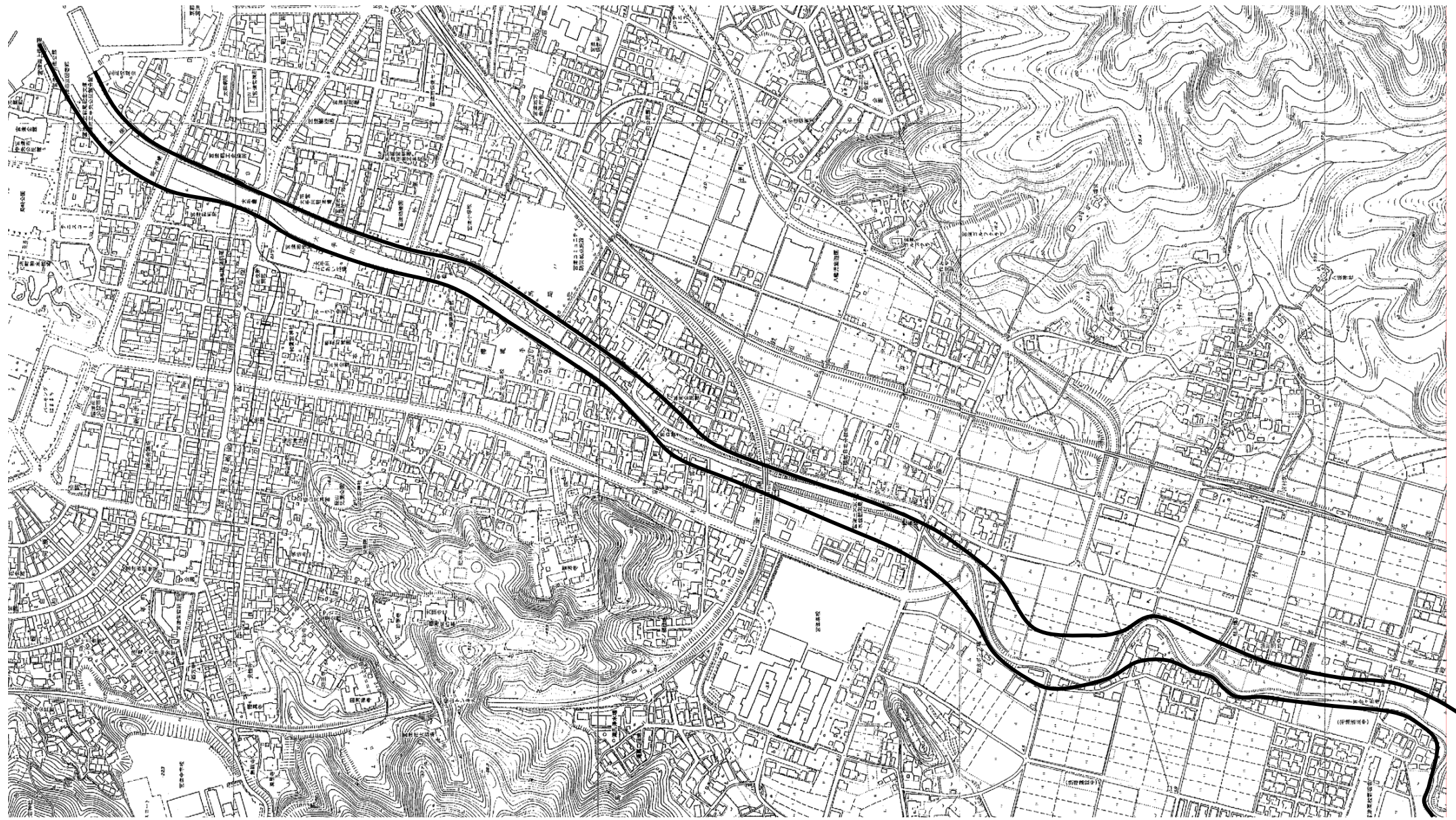
大手川平面図(その1) 縮尺1:5,000
