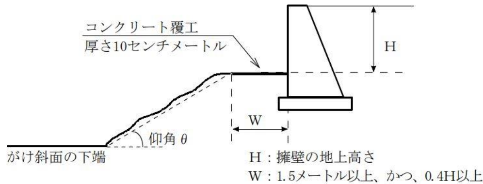
がけ斜面上に擁壁を設置する場合
