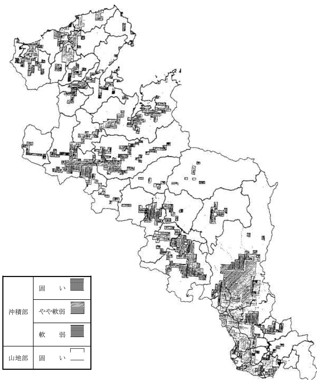
<地盤分類図>
