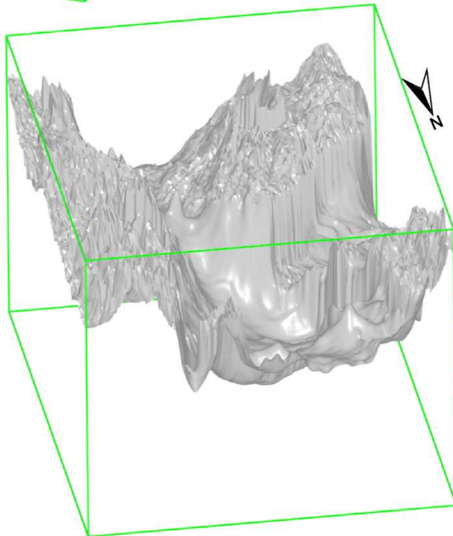
3次元地質モデル鳥瞰図 (基盤のみ、北北東より見て表示した図)
