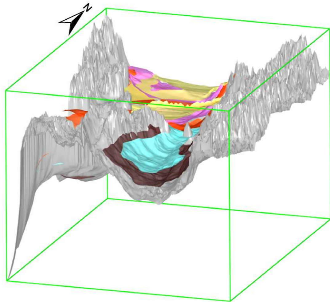
3次元地質モデル鳥瞰図 (南南東より見て表示した図)
