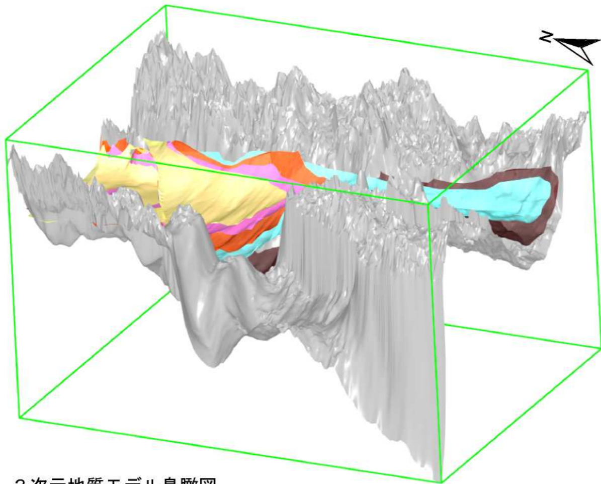
3次元地質モデル鳥瞰図 (西南西より見て表示した図 大阪平野側の層序は表示していない)
