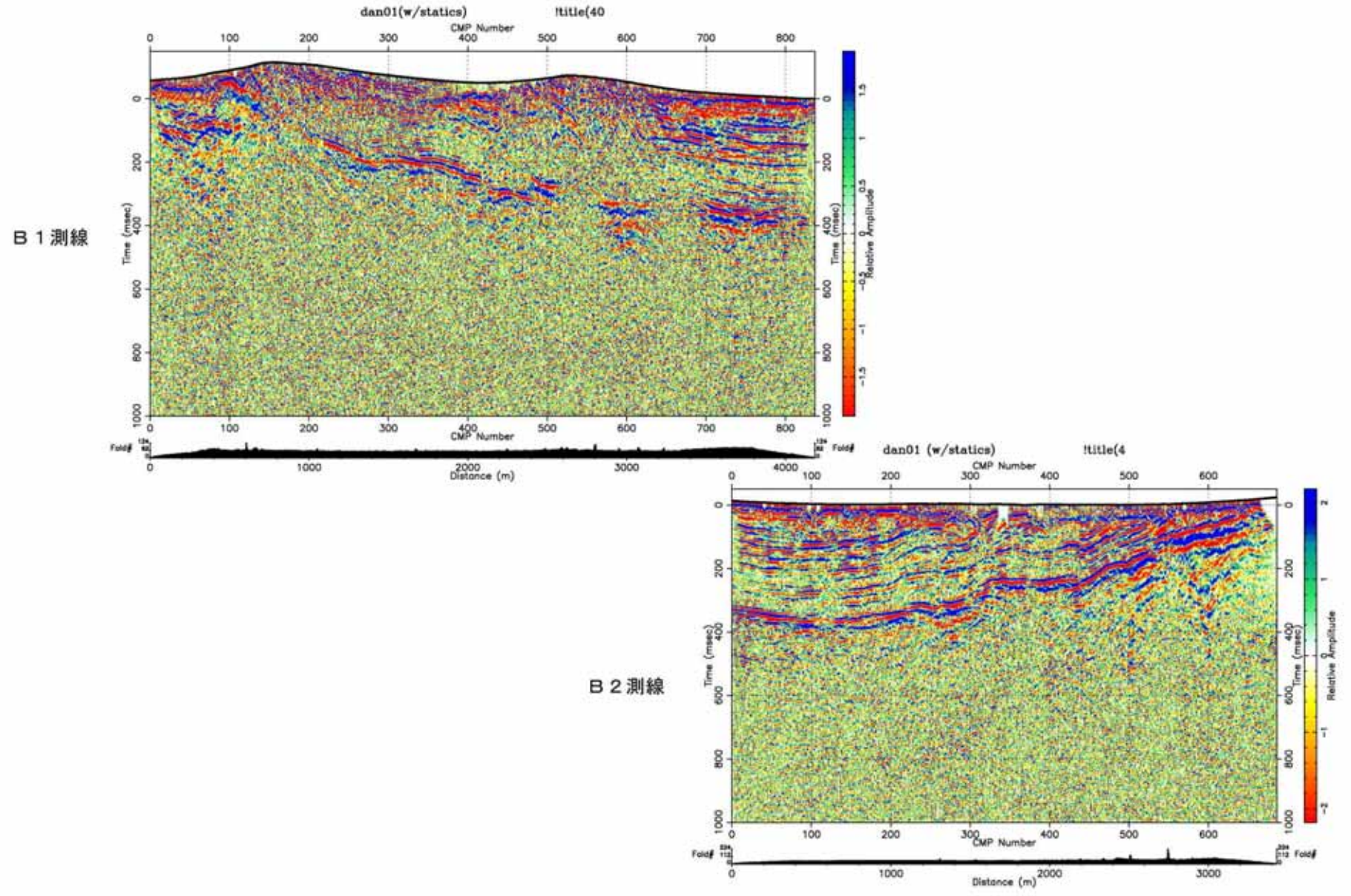
図-9 重合後時間断面（静補正までの波形処理を実施；処理途中） 縮尺1/25,000
