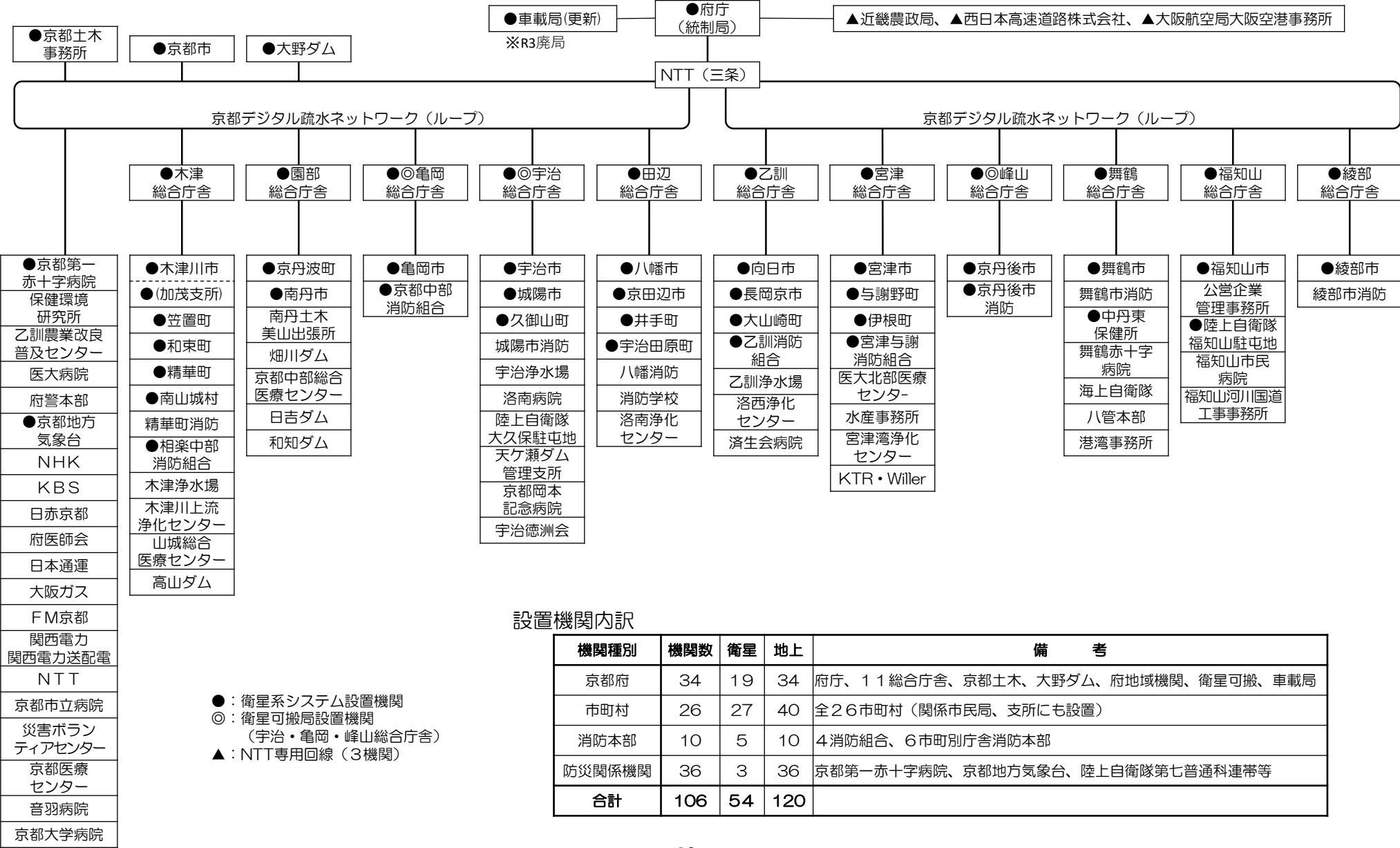
資料 2 - 3 京都府衛星通信系防災情報システム構成図 令和 6 年 4 月現在（平成 1 5 ～ 1 8 年度整備）
