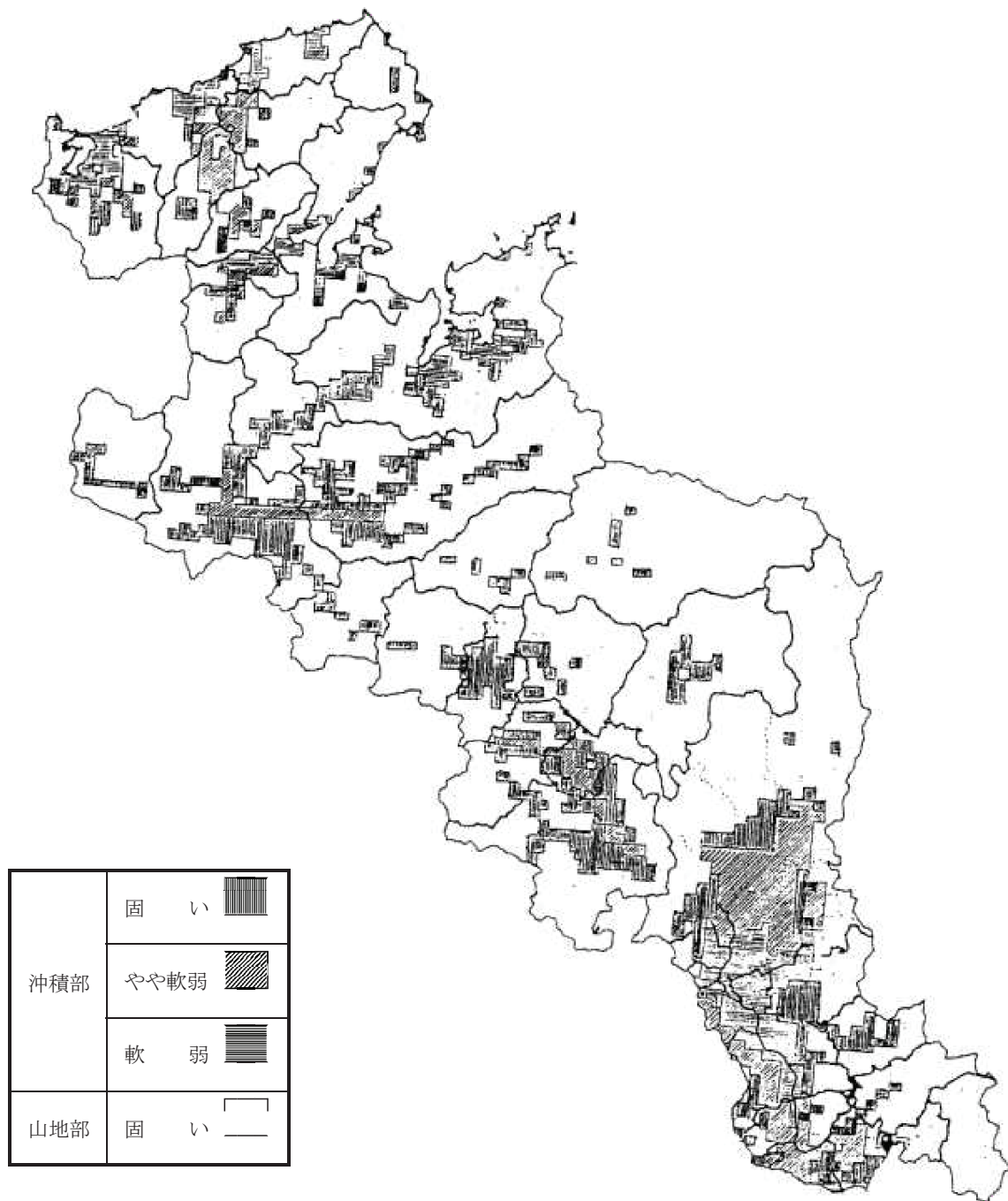
<地盤分類図>
