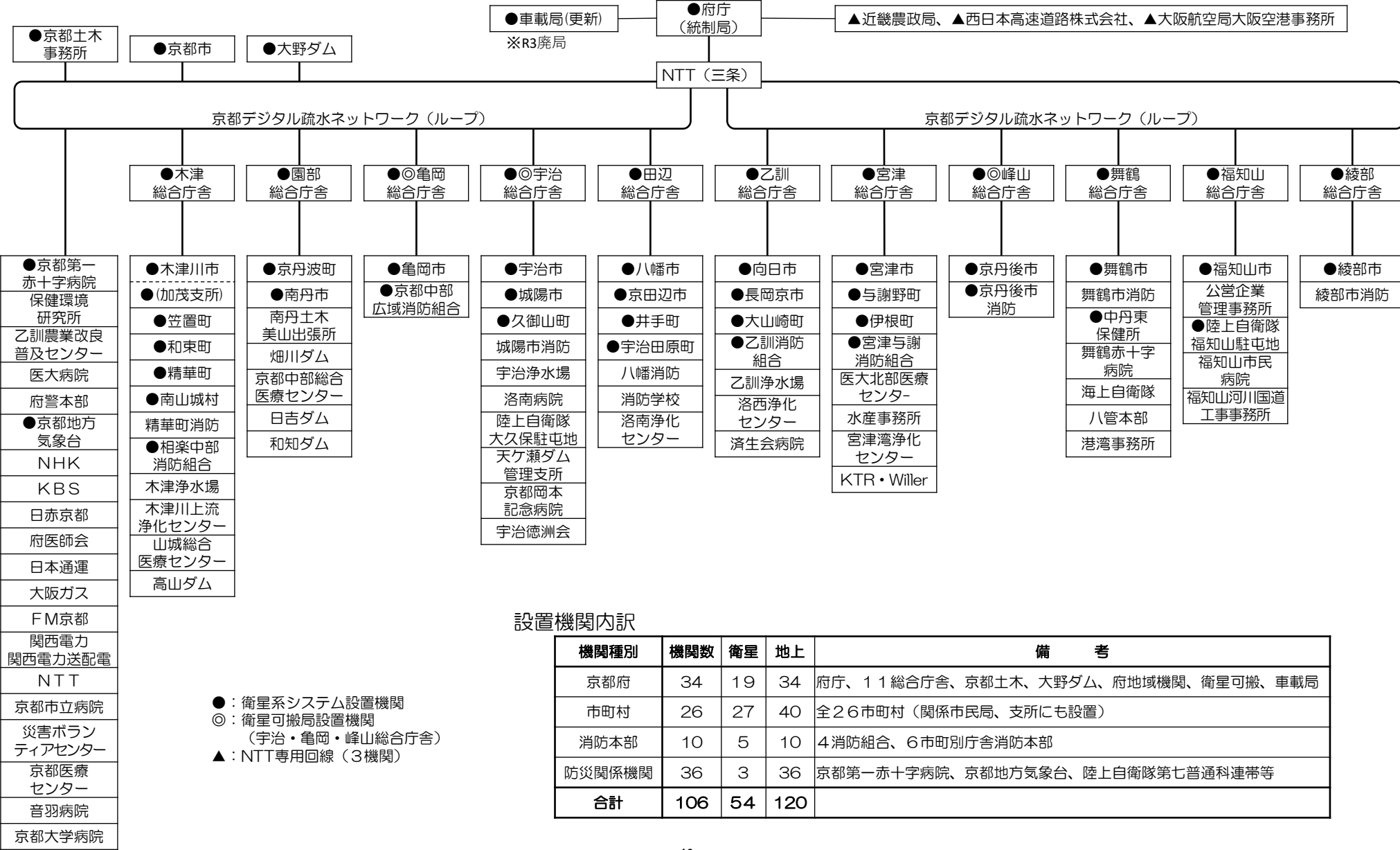
資料 2 - 3 京都府衛星通信系防災情報システム構成図 令和 7 年 4 月現在（平成 1 5 ～ 1 8 年度整備）
