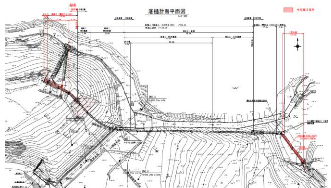
【計画平面図】
