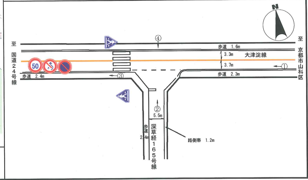
交差点図面
