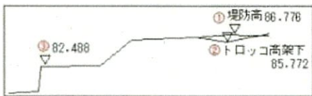
横断面
