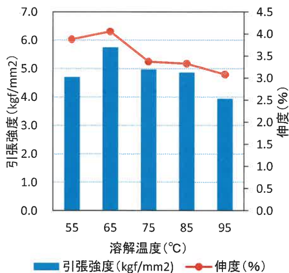
図 2 溶解温度とフィルムの強伸度
