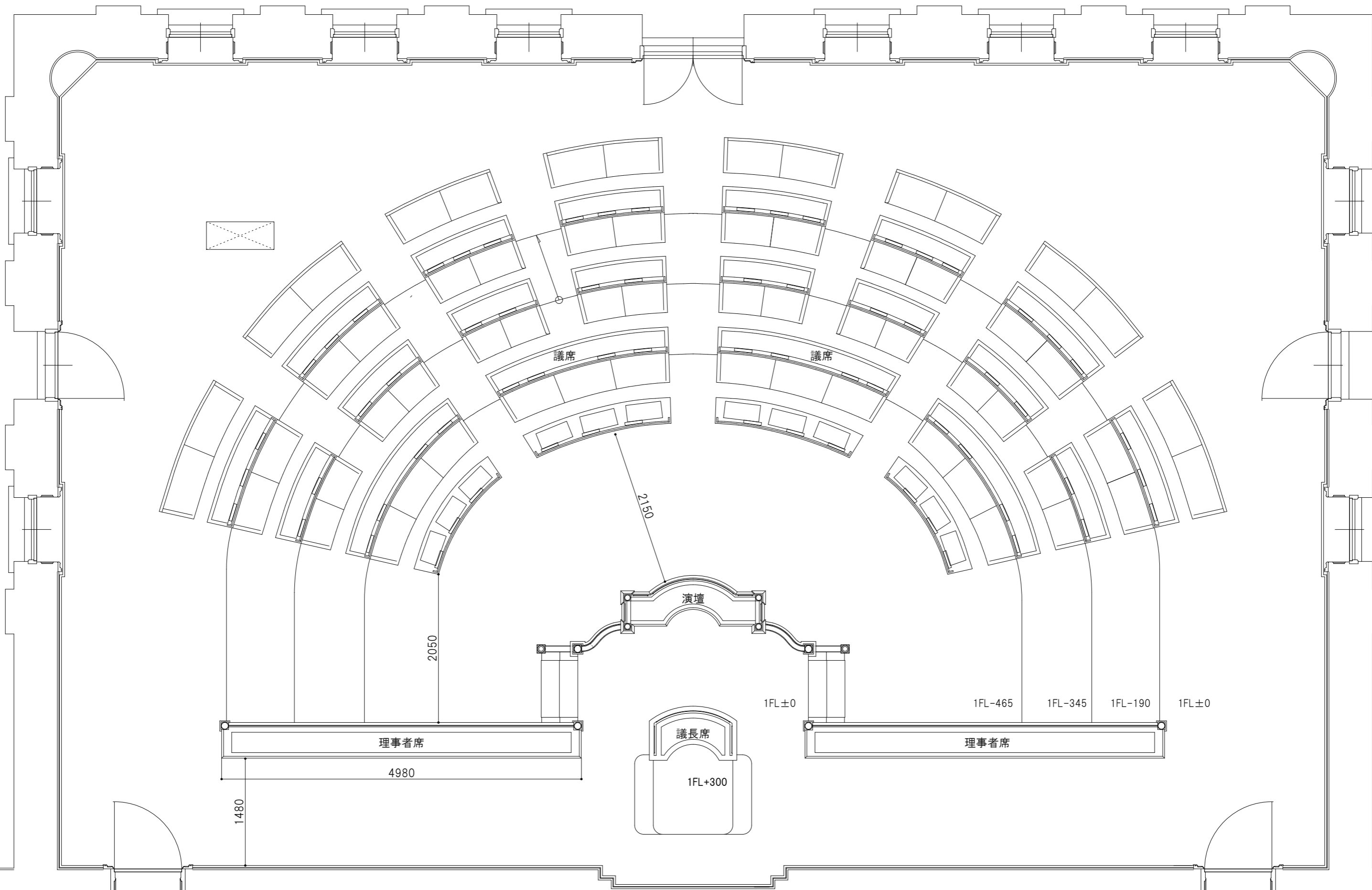
旧議場1階平面図 S:1/50(A3)
