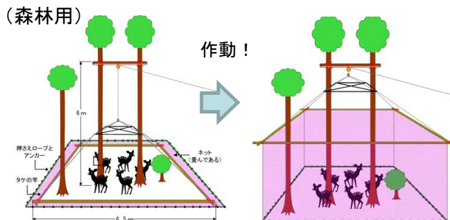
図3 新たに考案した遠隔操作型の森林用アップネット
