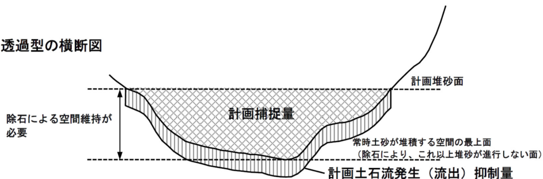
図 2-3 (1) 砂防堰堤の型式別の計画で扱う土砂・流木量等 (砂防基本計画策定指針（土石流・流木対策編）解説(H28.4) 第4節 4.3.1.1<解説>)
