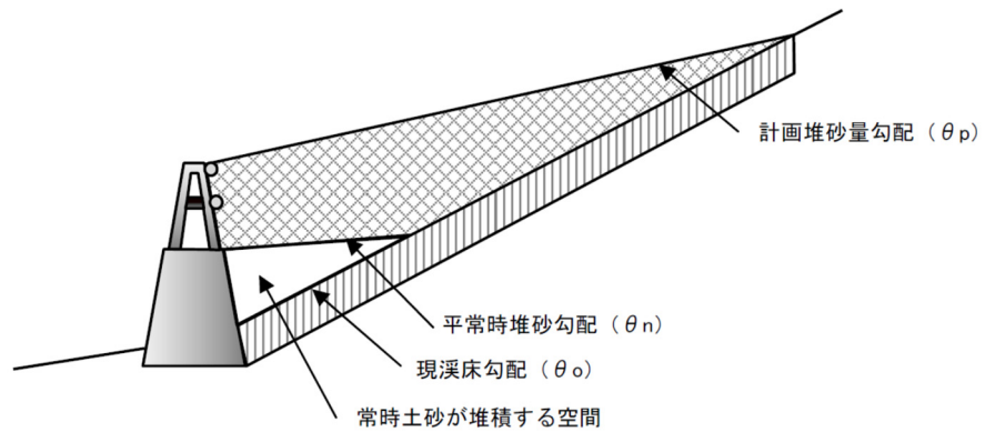
図 2-3 (2) 砂防堰堤の型式別の計画で扱う土砂・流木量等 (砂防基本計画策定指針 (土石流・流木対策編) 解説(H28.4) 第4節 4.3.1.1<解説>)
