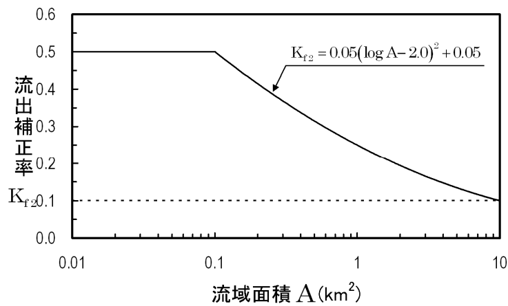
図 3-4 流出補正率
