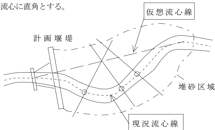
図 2-5 堆砂横断の方向
