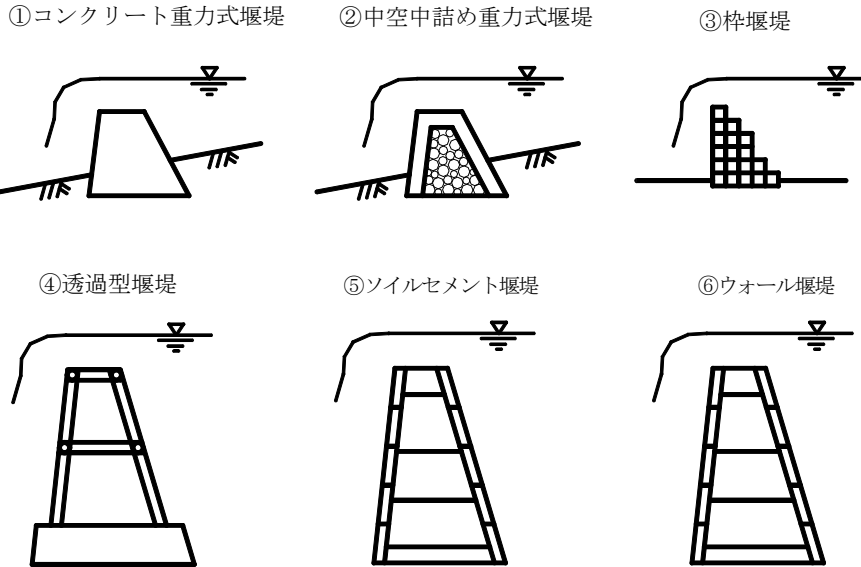
図 1-1 堰堤の設計理論による分類
