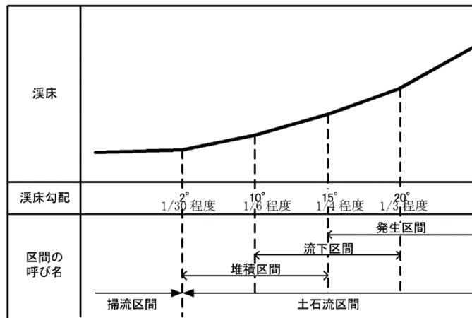
図 4-3 土石移動の形態の渓床勾配による目安 1)
