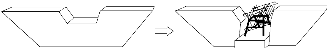
図 2-8 堰堤のスリット化
