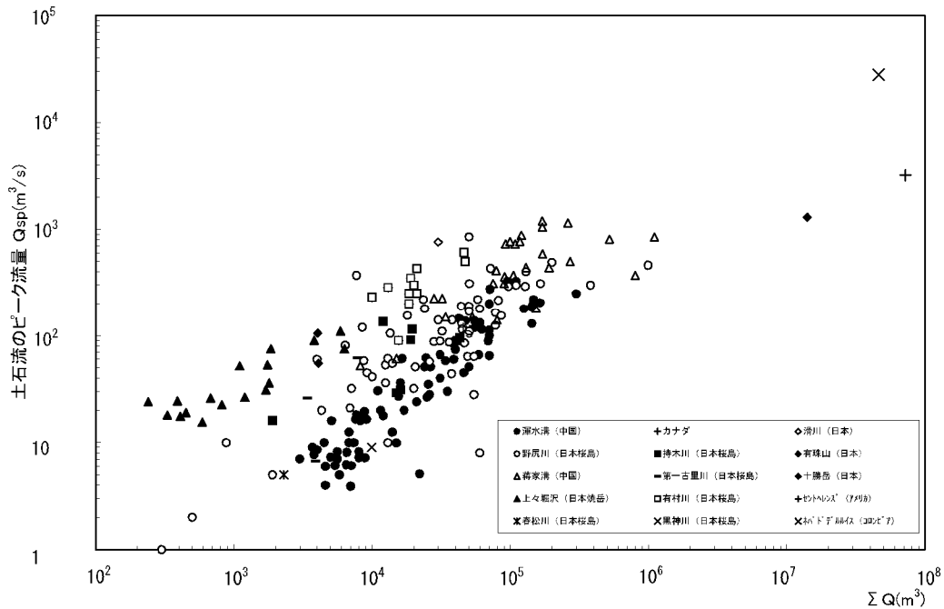
図 2-16 ピーク流量の相関 1) (原著ではΣQは Q_T と標記されている) (砂防基本計画策定指針 (土石流・流木対策編) 解説(H28.4) 第2節 2.6.3<解説>)
