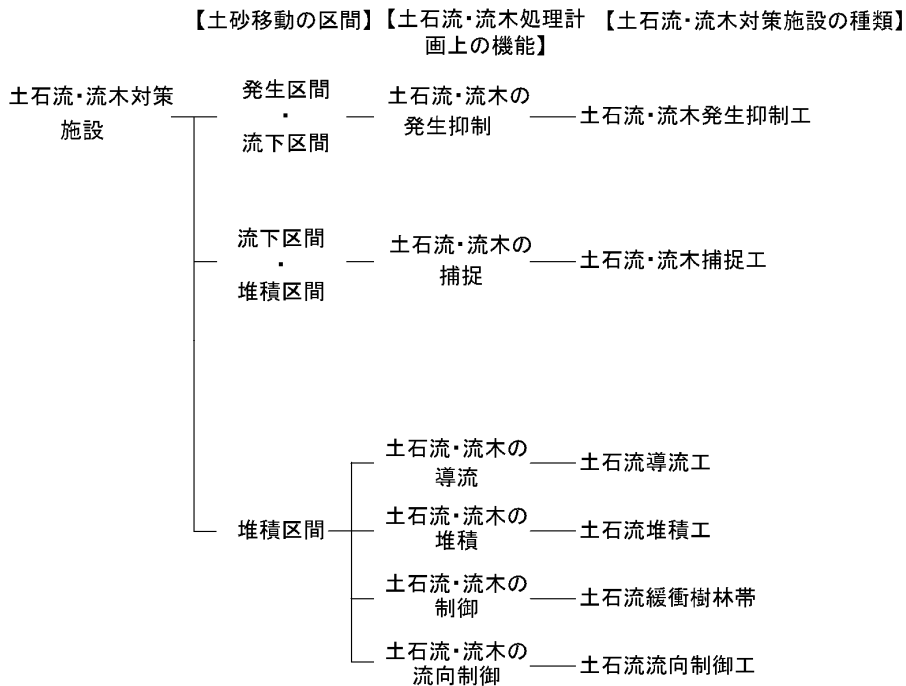
図 2-1 土石流・流木対策施設の種類の種類
