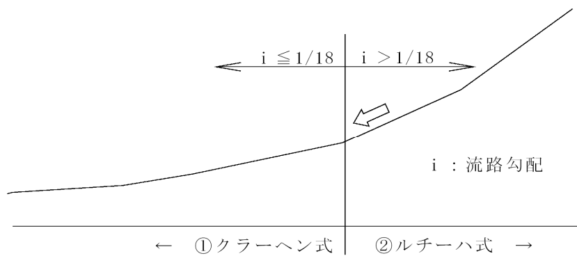
図 3-6 クラークヘン式とルチャーハ式の適用範囲
