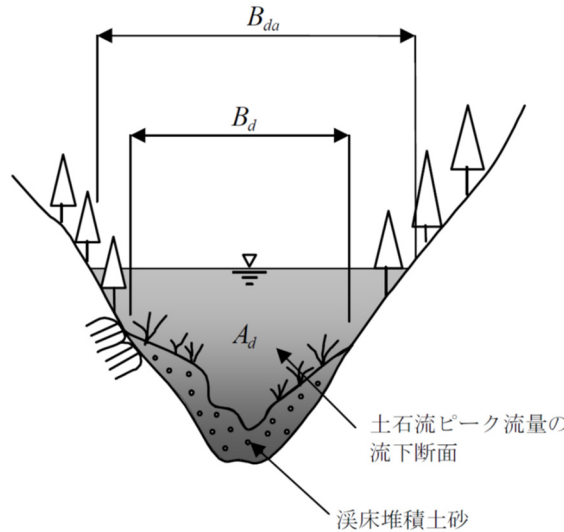
図 2-18 土石流の流下断面と流れの幅B da のイメージ
