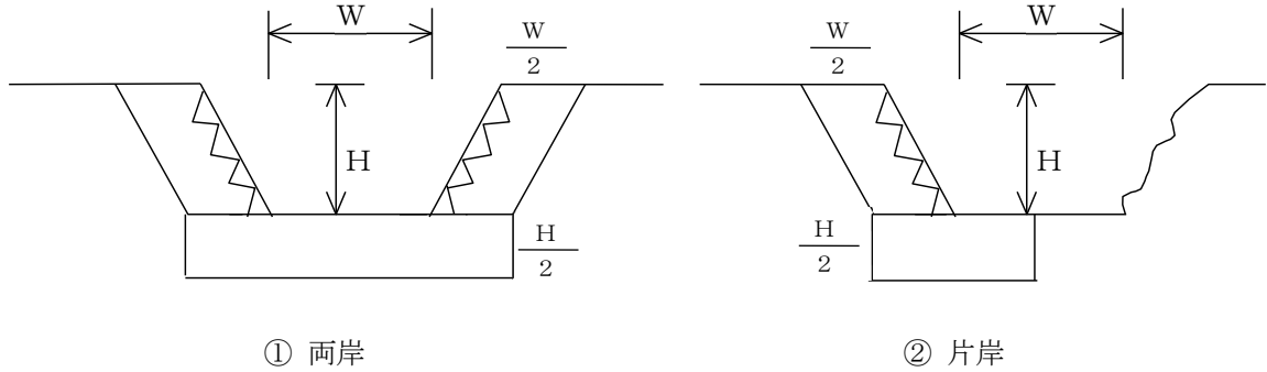
図 4-6 溪流保全工（流路工）の抑制土砂量
