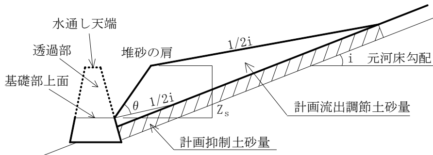
図 4-11 土砂調節のための透過型堰堤における計画流出調節土砂量の考え方
