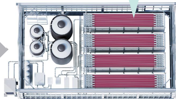
微生物培養プラント （京都大学内に4,000ℓ級を設置）
