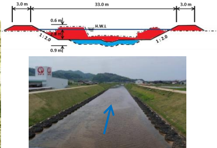
河道拡幅後の福田川
