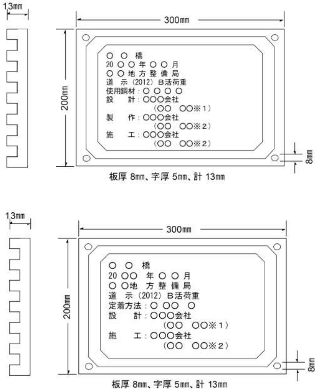
図 3-2-2 銘板の寸法及び記載事項
