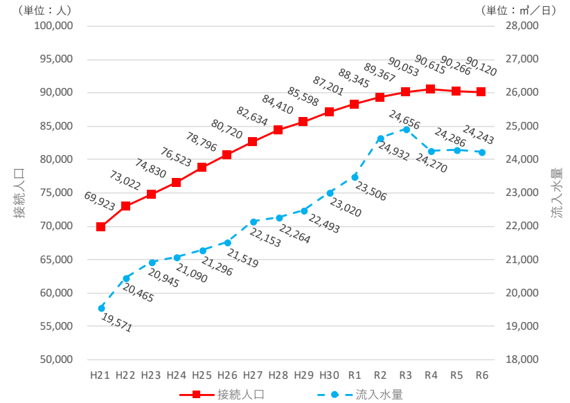
図 4.2 接続人口と流入水量の推移 (木津川上流流域下水道)
