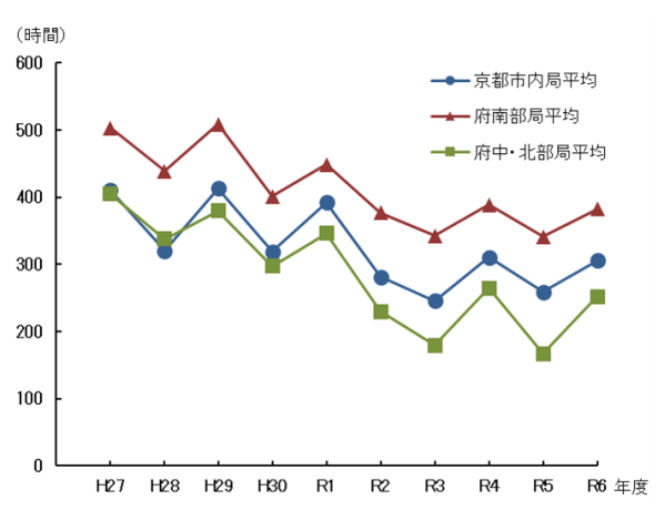
光化学オキシダント環境基準(0.06ppm)超過時間数の経年変化
