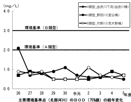
主要環境基準点のBODの経年変化(左:南部河川、右:北部河川)
