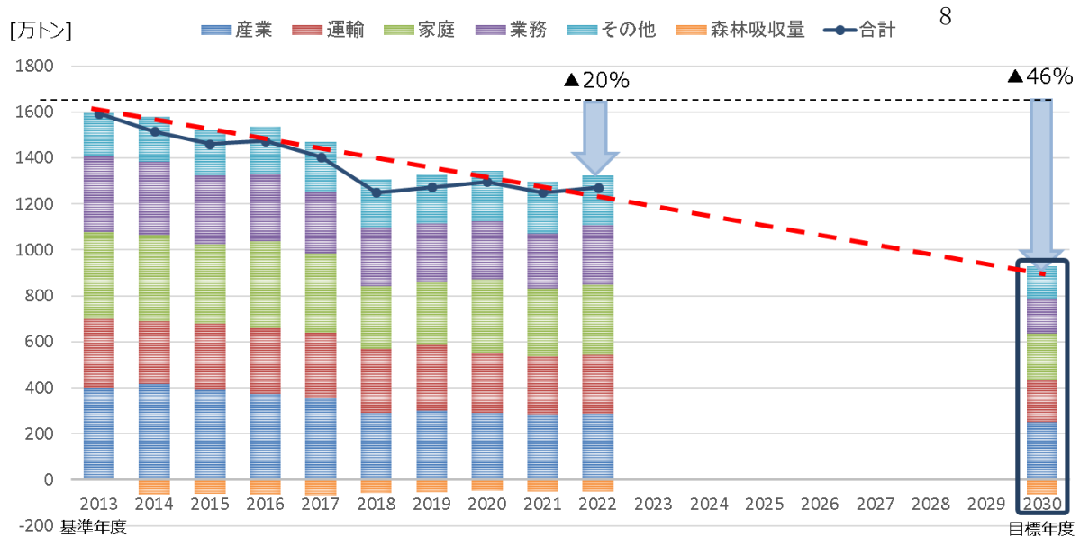
9 温室効果ガスの総排出量の推移
