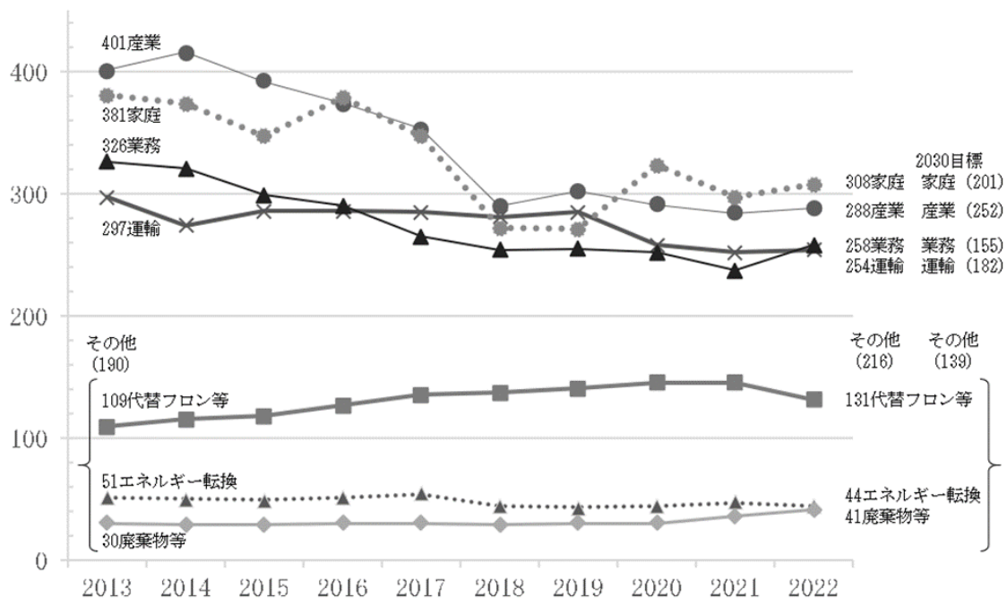
9 温室効果ガスの総排出量の推移
