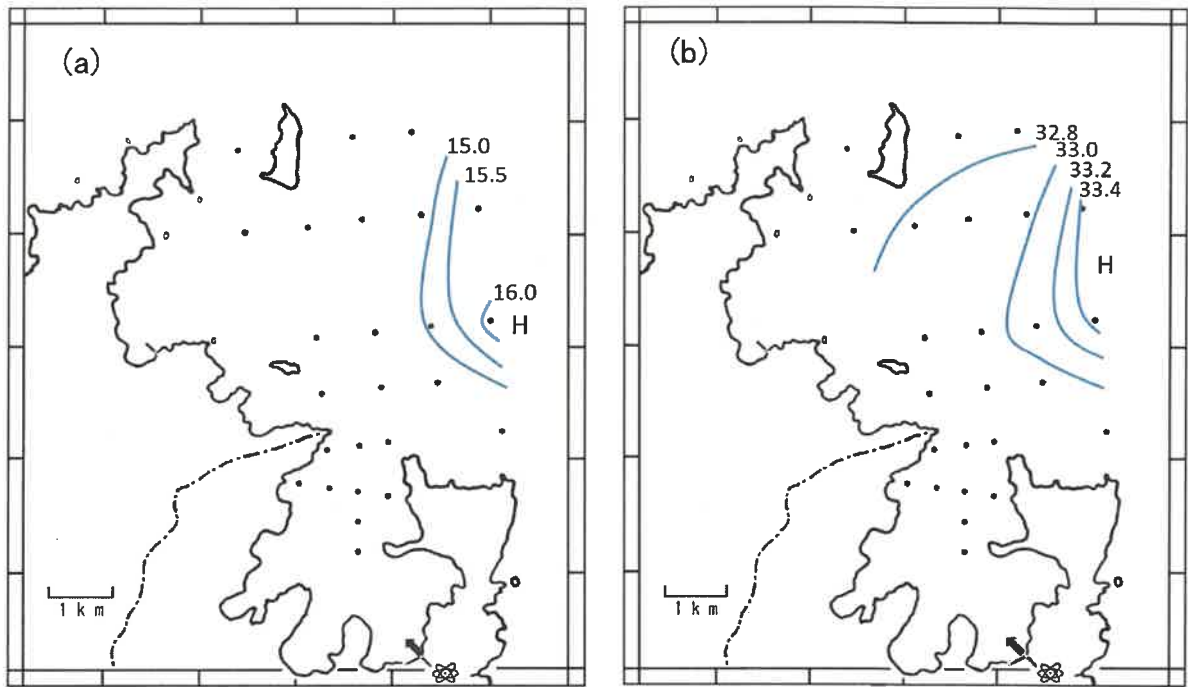
図2-5 表層水温(a)および表層塩分(b)分布図(令和2年12月)
