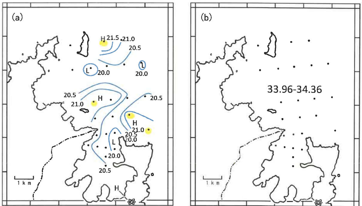
図2-2 表面水温(a)および表面塩分(b)分布図(令和2年6月)
