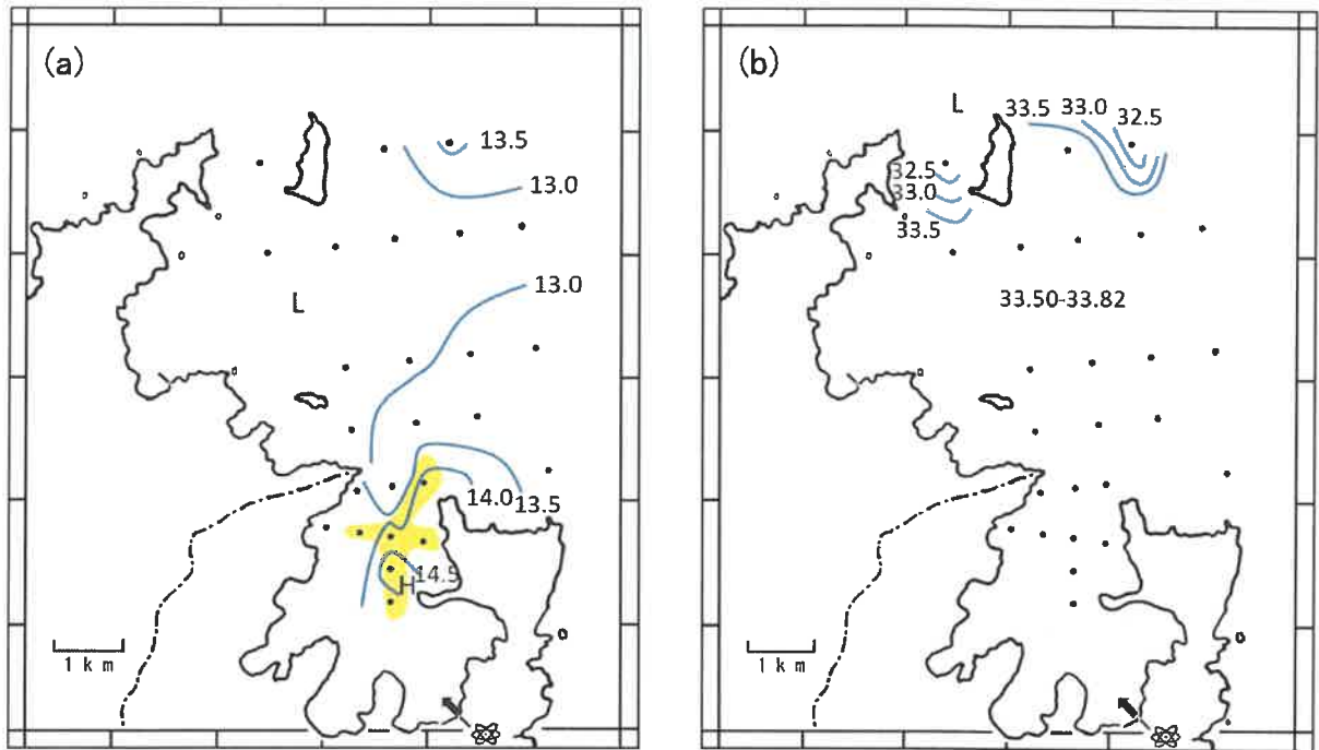
図2-1 表層水温 (a) および表層塩分 (b) 分布図 (令和2年4月)
