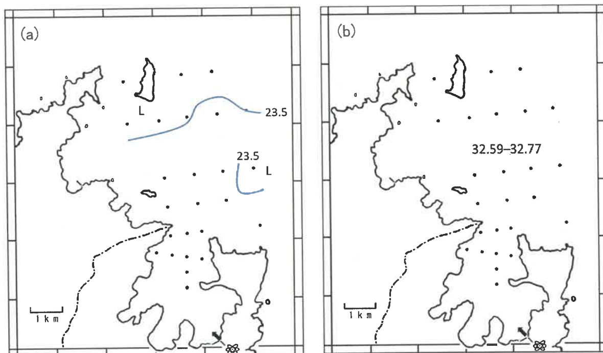
図2-4 表面水温(a)および表面塩分(b)分布図(令和2年10月)
