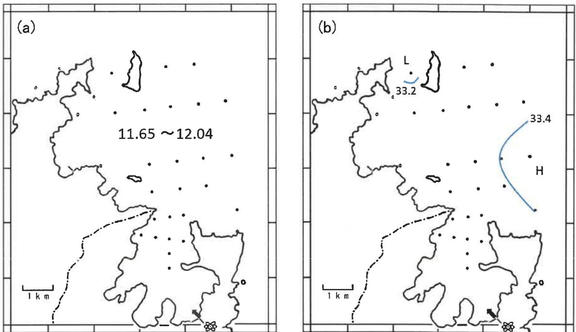
図2-6 表層水温(a)および表層塩分(b)分布図(令和3年2月)
