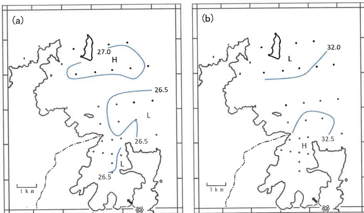
図2-3 表面水温(a)および表面塩分(b)分布図(令和2年8月)
