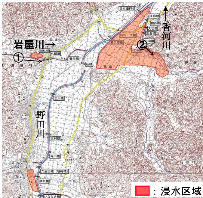
図 5 浸水被害状況 (平成 10 年 9 月台風 7 号)
