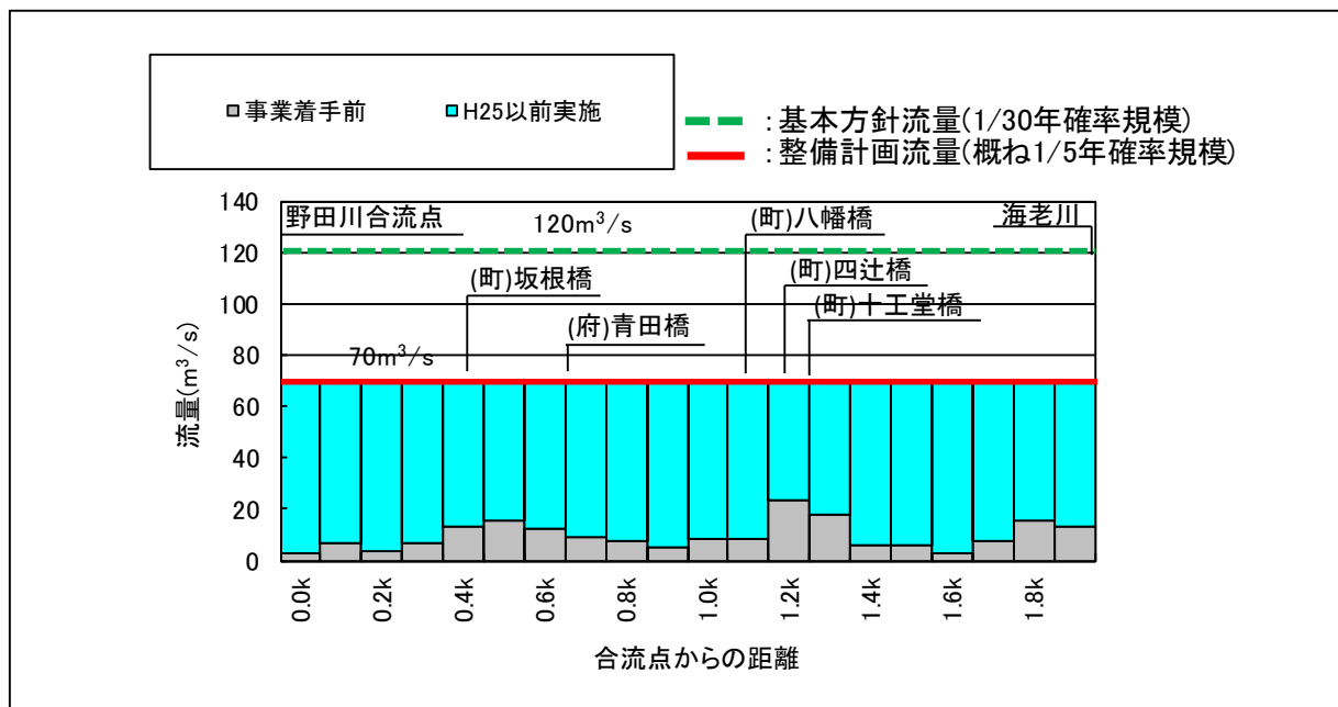
図 1 1 岩屋川流下能力図
