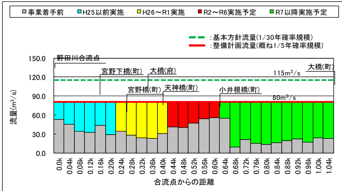
図 1 2 加悦奥川流下能力図
