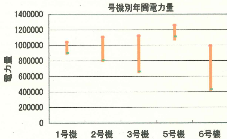
1号機～6号機（4号機を除く）の年間電力量
