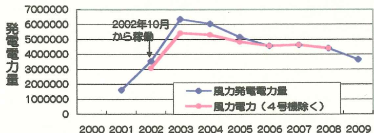
1号機～6号機（4号機を除く）の発電電力量の推移
