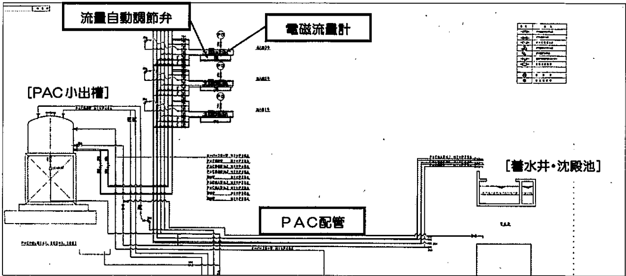
(2) 木津浄水場 PAC 注入設備系統図
