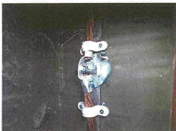
③ 避雷導線の接続
