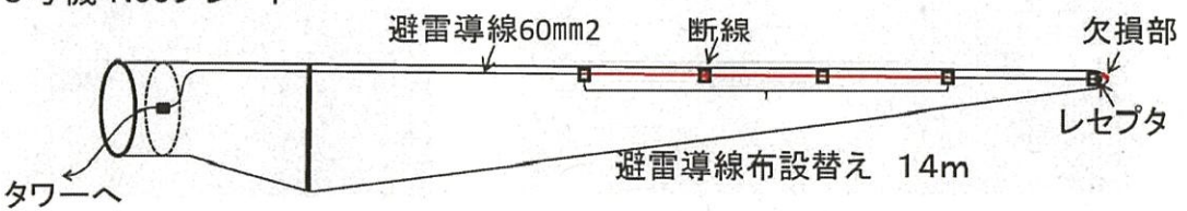
風車6号機 No3ブレード
