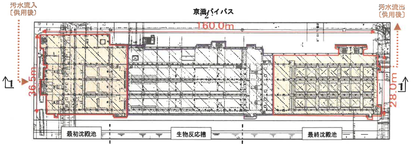
[E1系 平面図]
