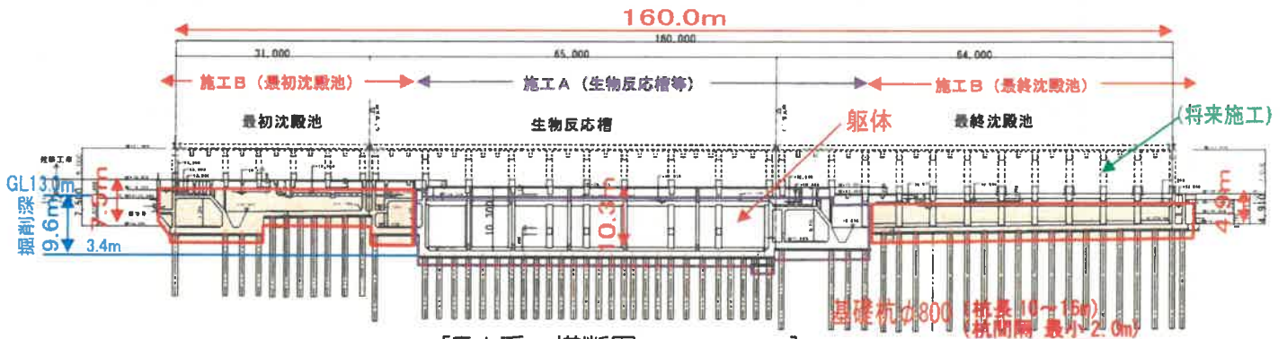
[E1系 横断図 (1-1断面)]
