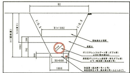
【パイプ埋設標準断面図】
