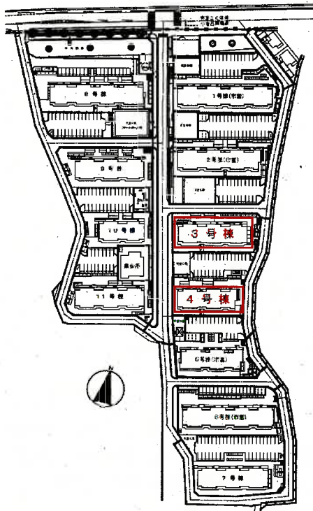
府営住宅白鳥団地 全体配置図
