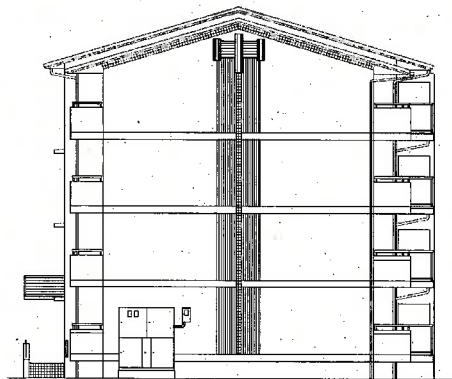
3号棟 立面図 西面
