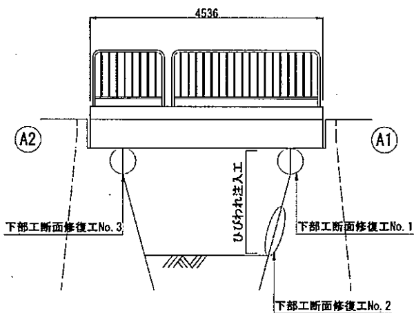
<補修計画図>
