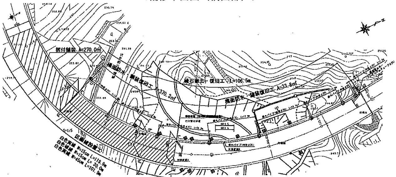
<補修平面図 (上部工下面部: コンクリート剥落対策範囲)>
