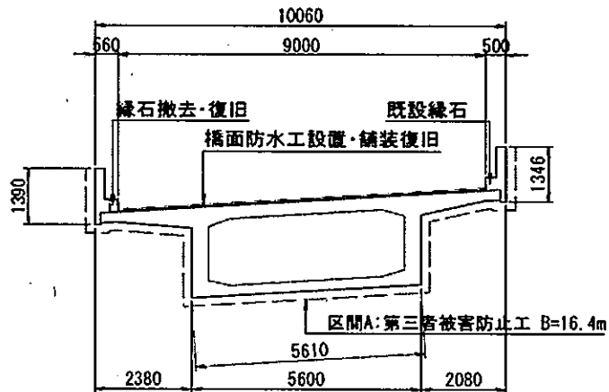
<横断面図>
