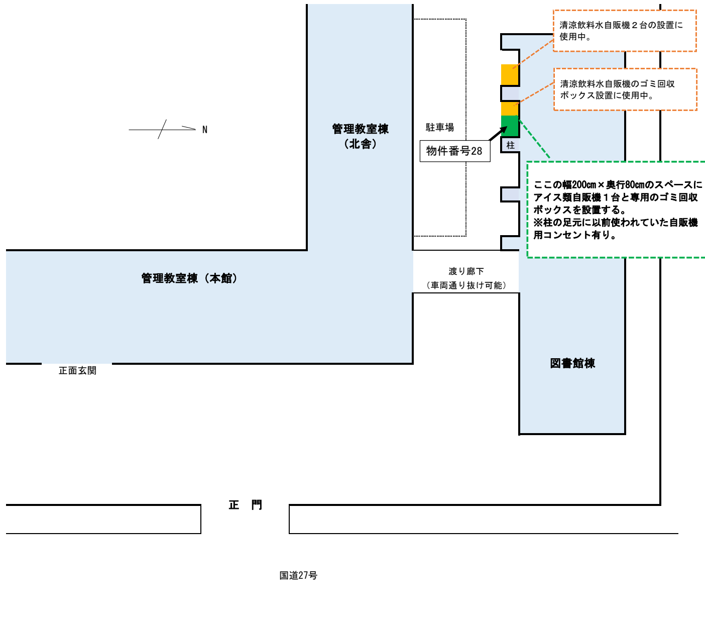
物件番号28 京都府立西舞鶴高等学校 アイス類自動販売機設置位置の見取り図
