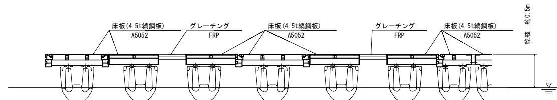
断面図
