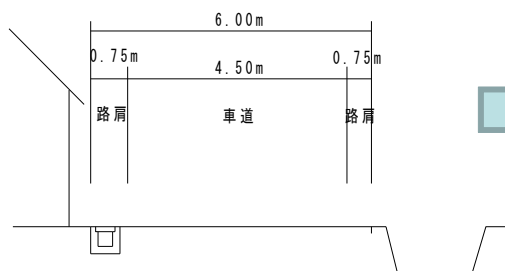
現道 断面図
