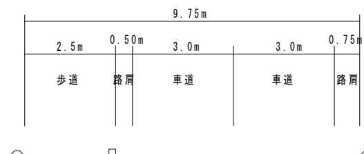
バイパス 標準断面図
