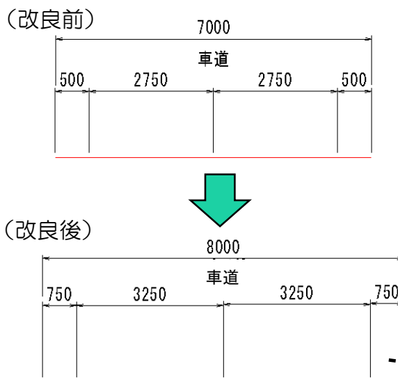
【標準横断図】
