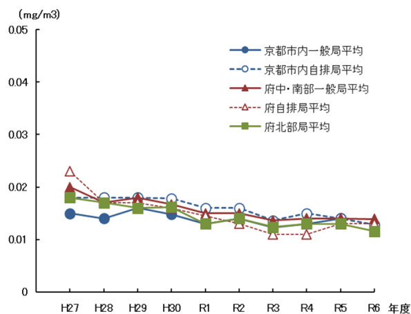
浮遊粒子状物質年平均値の経年変化
