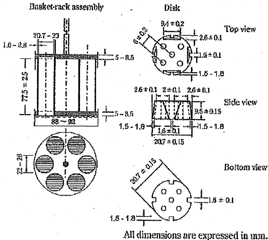
Fig. 6.09-1 Disintegration apparatus
