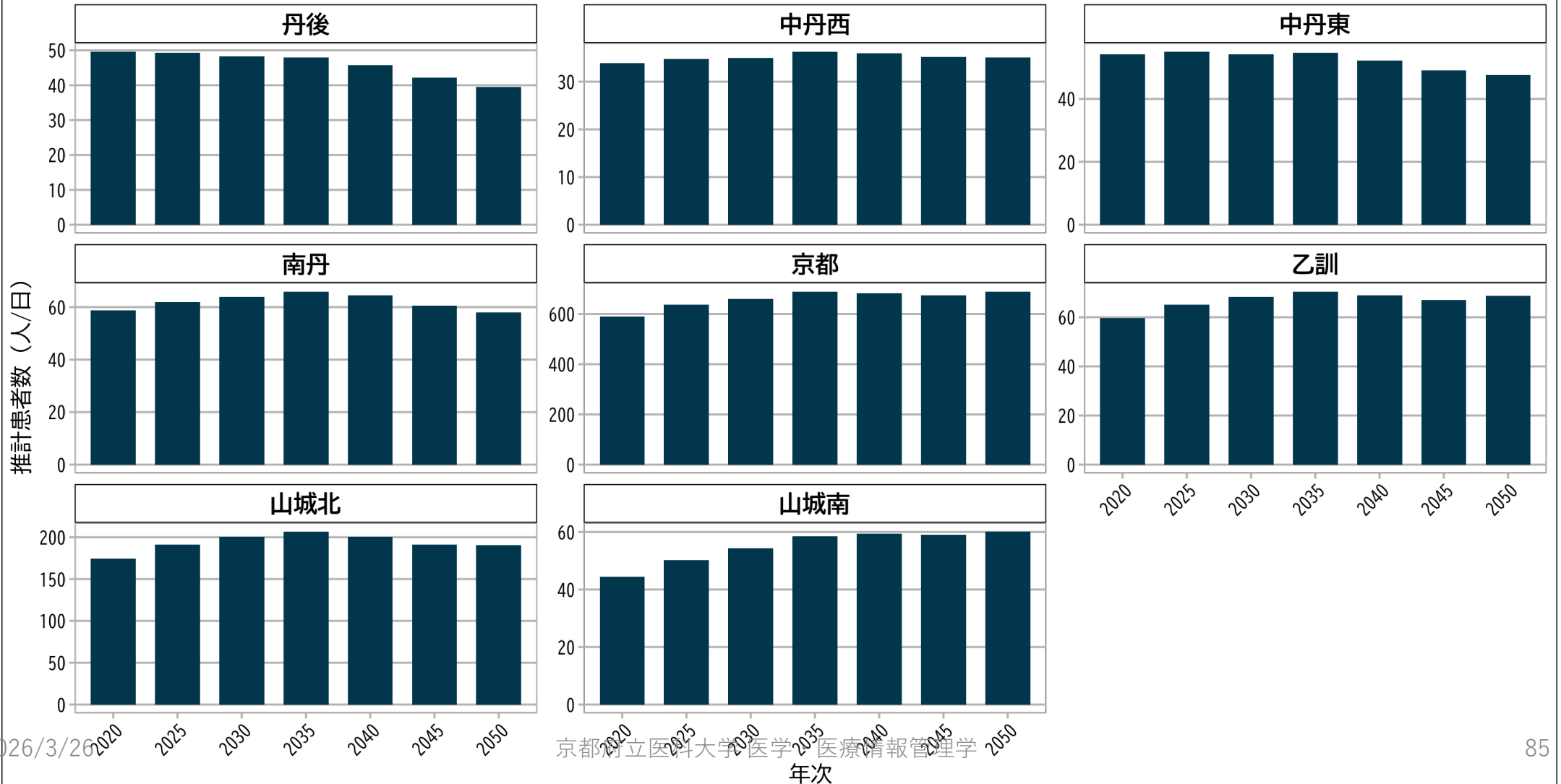
医療圏別 将来入院患者数の推移（腎尿路生殖器系の疾患） 2020年-2050年 / 各医療圏でY軸のスケールが異なる点に注意
