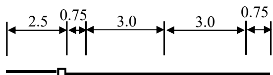
標準横断
