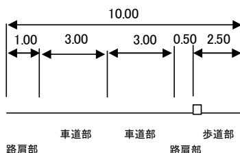
標準断面図(改良前)
