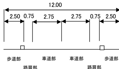
標準断面図(改良後)
