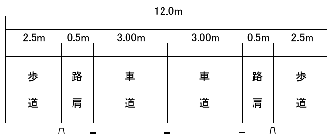
標準横断面
