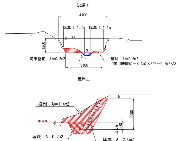
標準断面図
