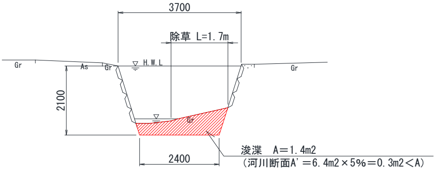
標準断面図
