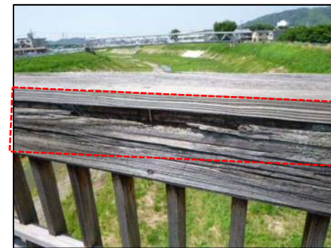
高欄の損傷
