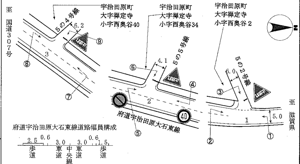
交差点図面
