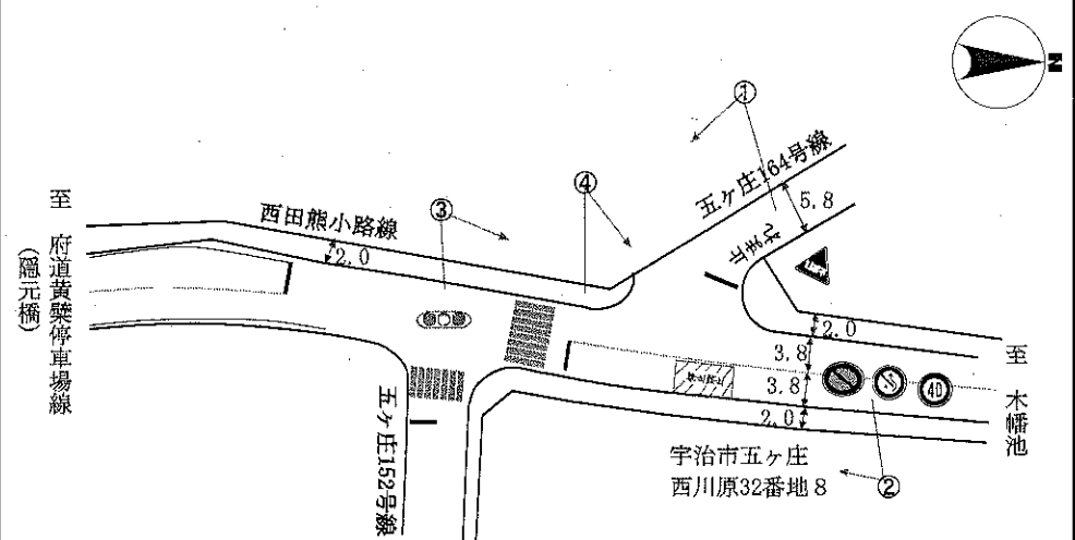
交差点図面
