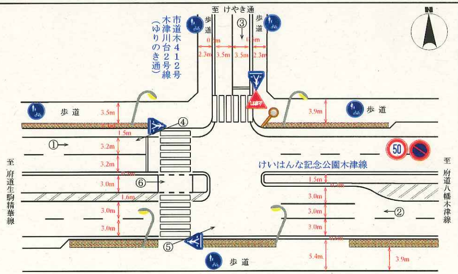
交差点図面
