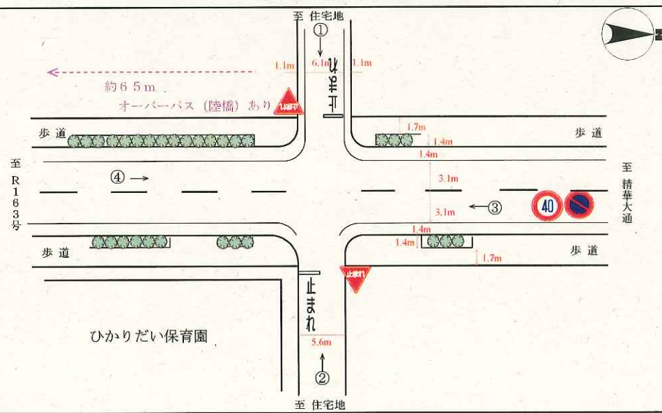
交差点図面
