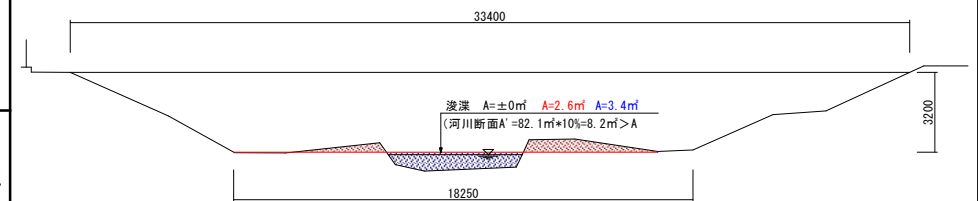
標準断面①
