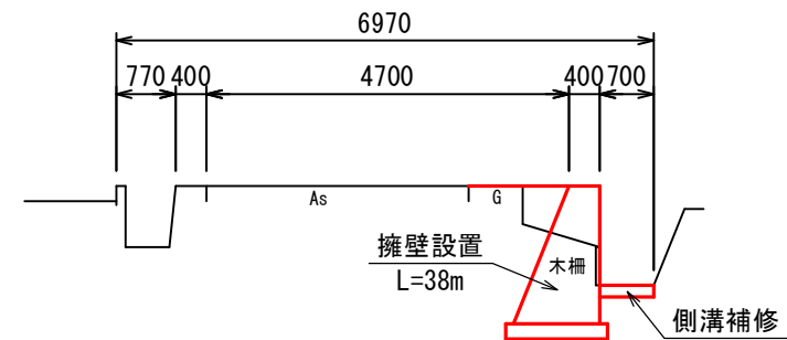
標準断面図
