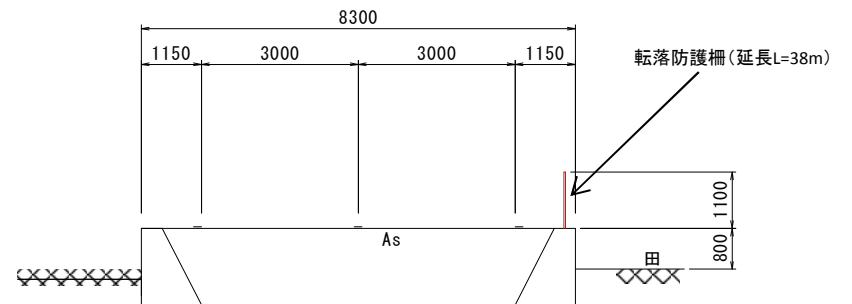
標準断面図(単位: mm)
